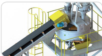
Alimentação com esteira transportadora. Feeding with conveyor system. Alimentación con cinta transportadora.
